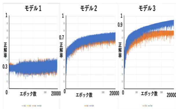
図1 学習曲線
